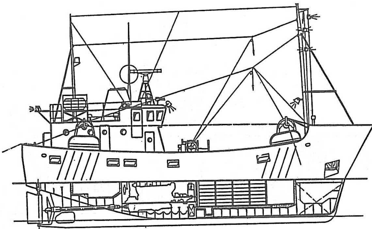
Sylwetka kutra serii KB-21
