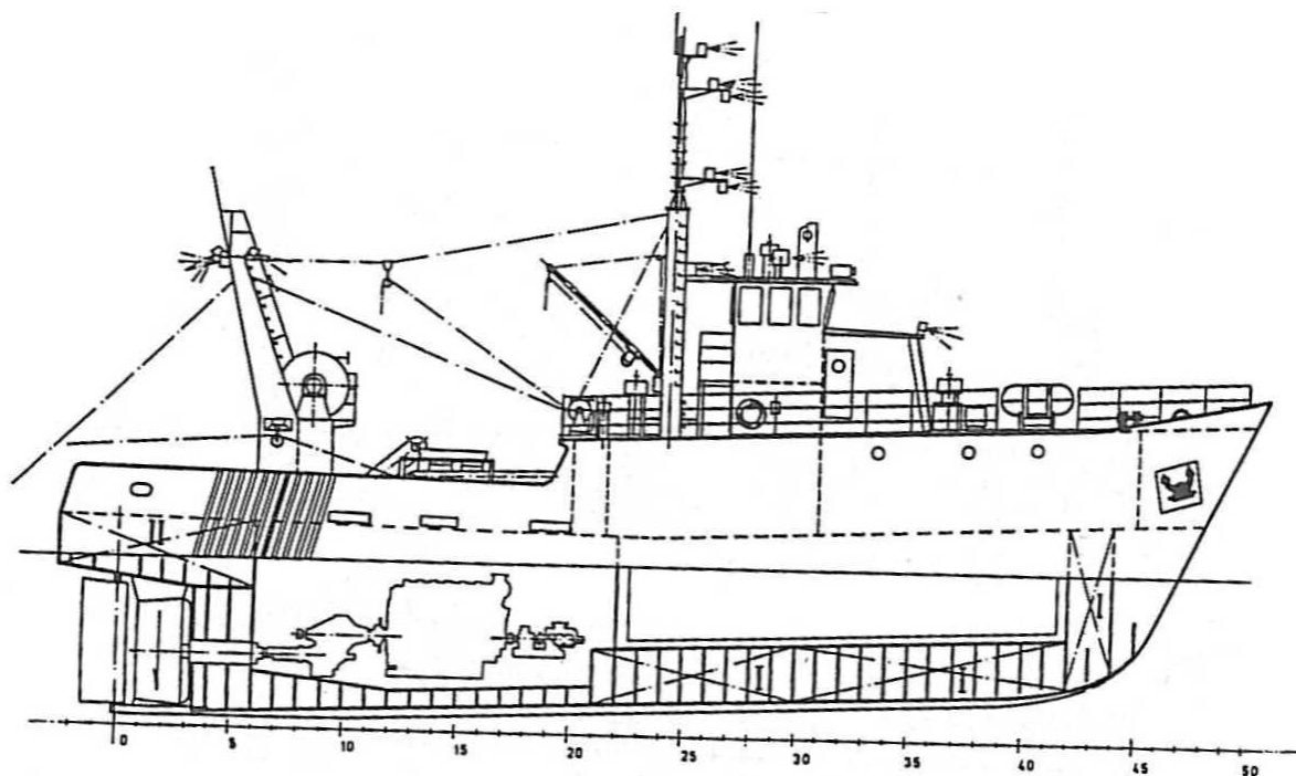
Sylwetka kutry typu B-280 budowanego w Ustce
